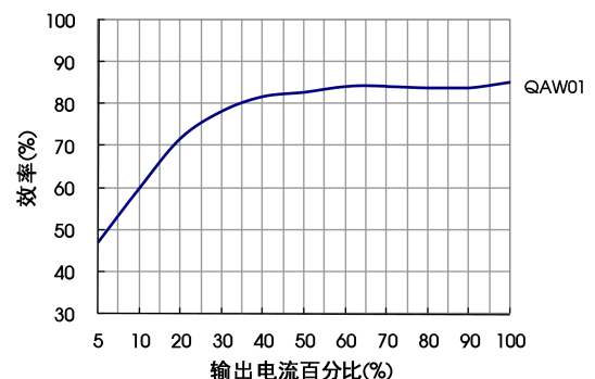
效率Vs输出负载(标称输入电压)
